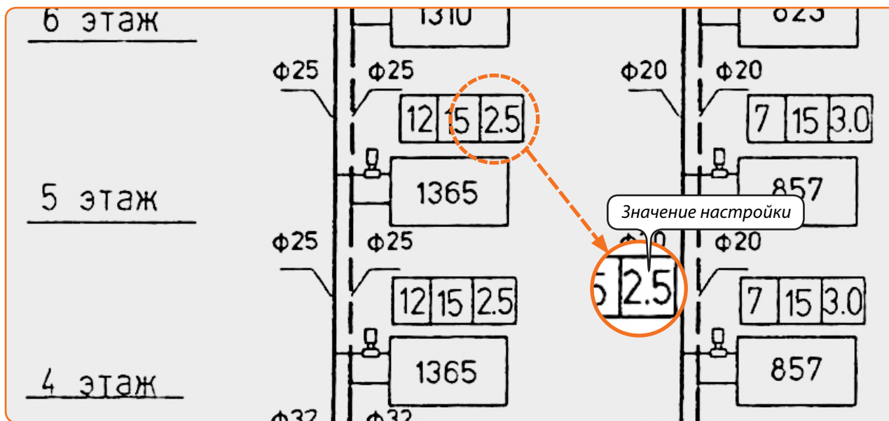
НАСТРОЙКИ КЛАПАНОВ. ПРИВЯЗКА К ПРОЕКТУ
