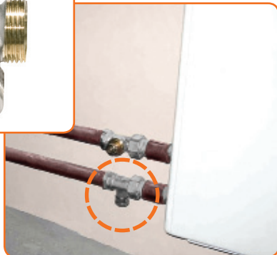
Клапан RLV
