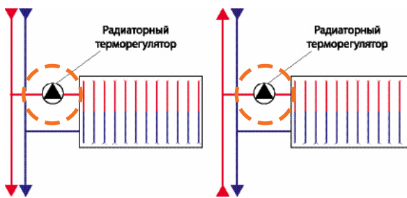
Рис. Б. Двухтрубная система отопления
