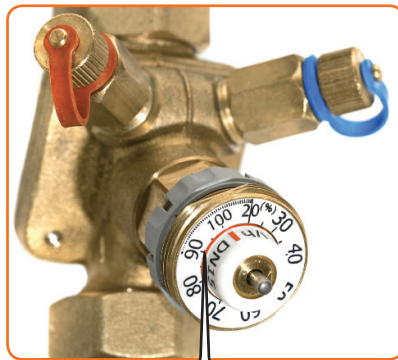
Настройка 100% (виден красный ободок)
